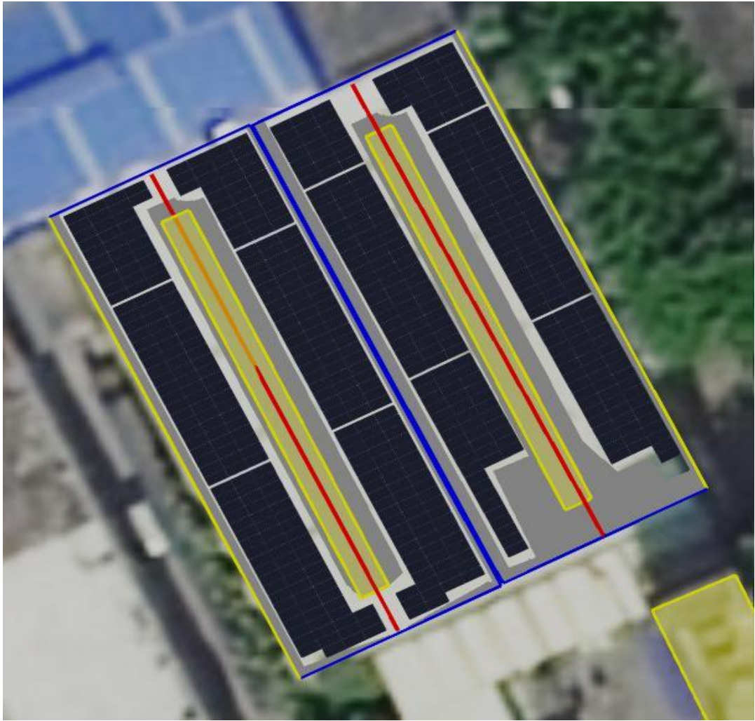
图 1-7 光伏布置图
